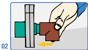
02 Introduzca la conexión en la boquilla macho hasta hacer tope. Cuando se haya cumplido el tiempo de calentamiento indicado en la tabla 2, retire la conexión de la boquilla y apóyela, sobre una superficie limpia, seca y a resguardo de corrientes de aire.
