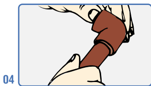
04 Transcurrido el tiempo de calentamiento retire el tubo e insértelo en la conexión sin pérdidas de tiempo.
