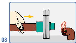
03 Introduzca el tubo en la boquilla, observando no sobrepasar la marca hecha previamente.
